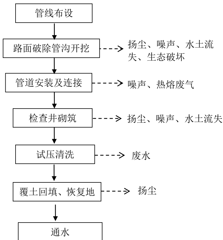
图 4-1 管网施工工艺流程及产污环节图
