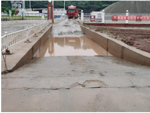
车轮清洗池
