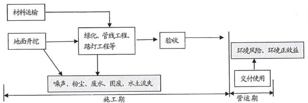
图 3-2 道路管网及配套设施施工工艺流程及产污流程图
