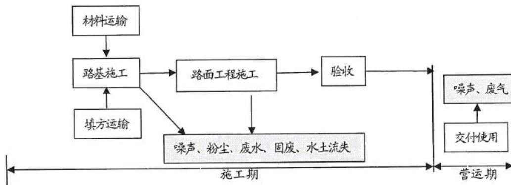
图 3-1 道路及配套设施施工工艺流程及产污流程图
