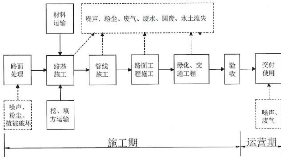
图 3-1 道路及配套工程施工流程及产污位置图
