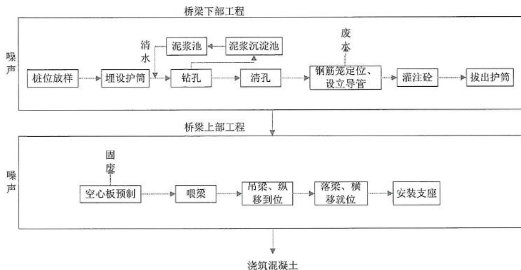
图 3-2 桥梁施工工艺流程及产污位置图
